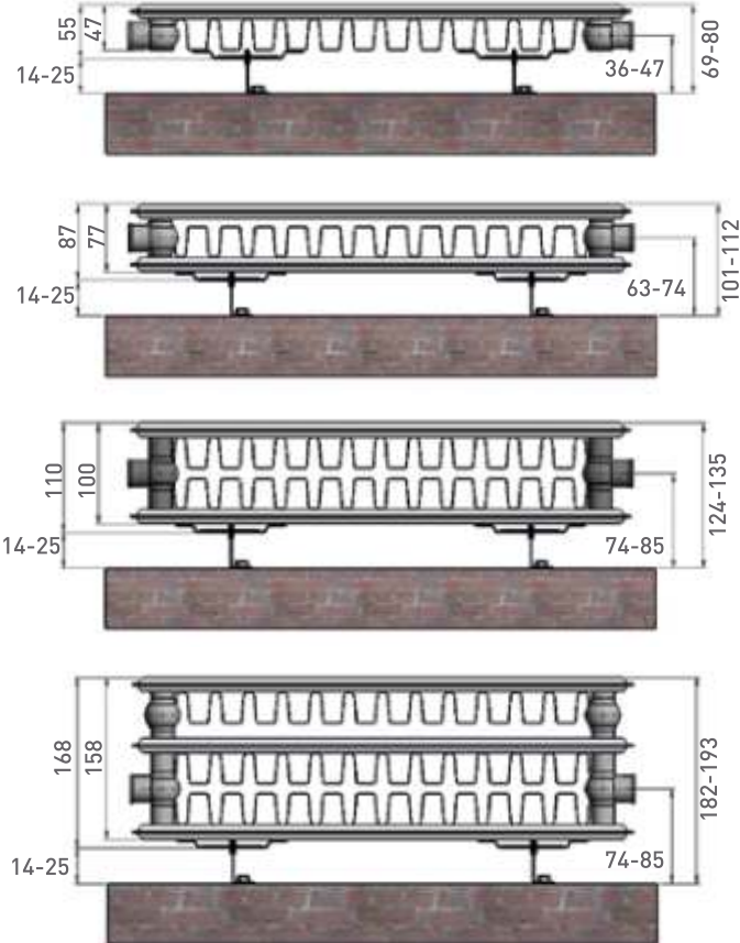
Klasik Radyatör Duvar Bağlantıları
