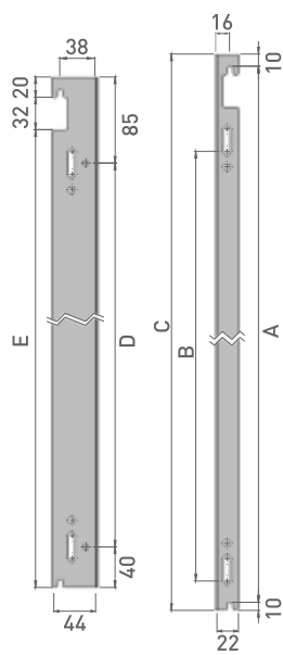
Dikey Radyatör Askıları
