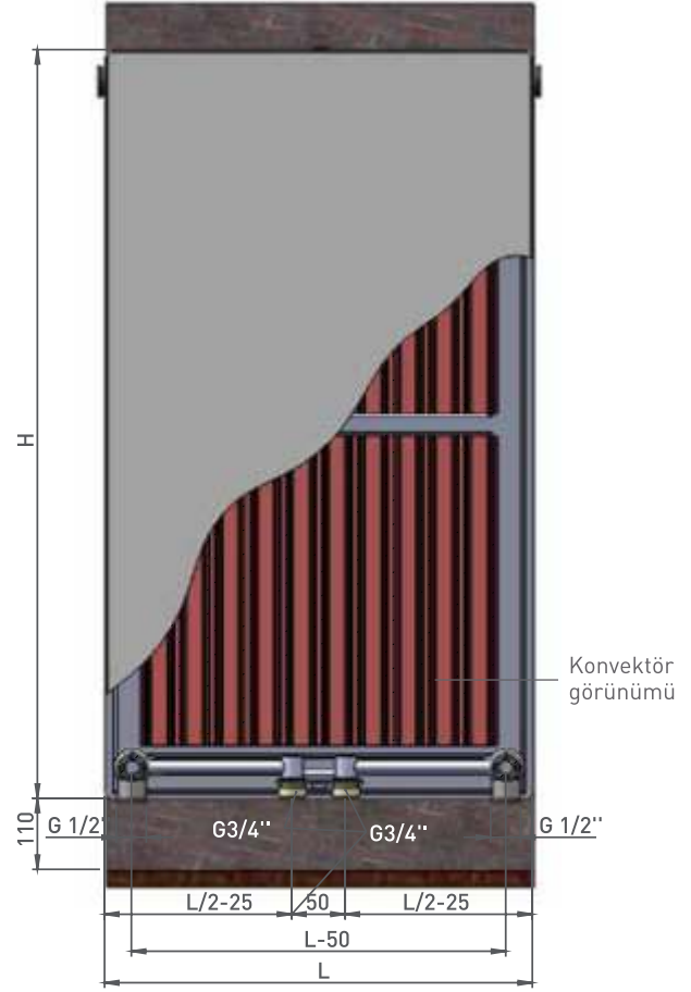
VK Radyatör Duvar Bağlantıları
