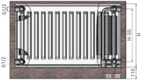
VK Radyatör Ön Kesit Görünümü
