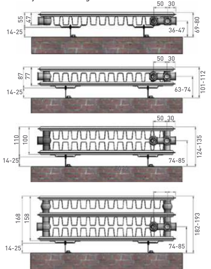
VK Radyatör Duvar Bağlantıları
